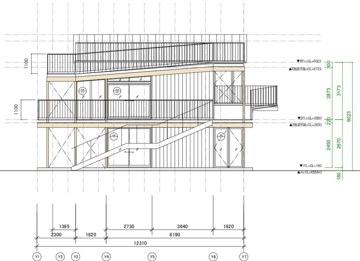
西側立面図
