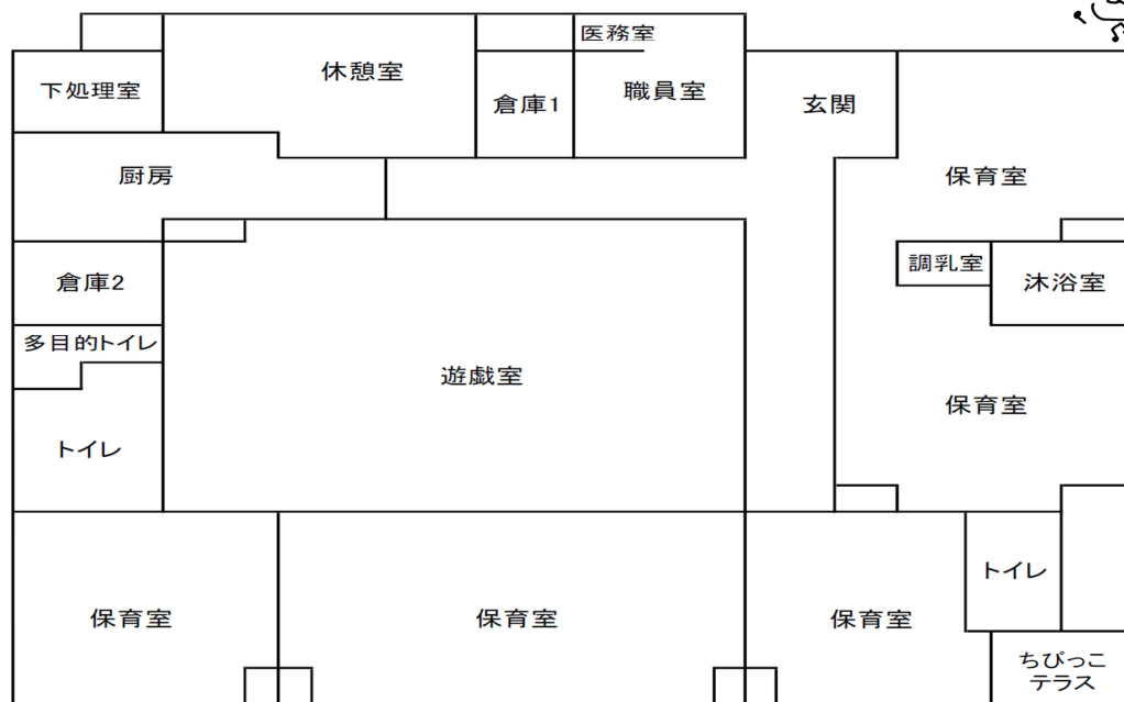
平面図
