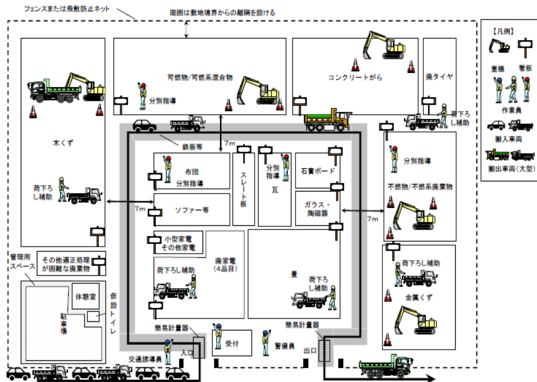
図 4-3 仮置場のレイアウトの例
